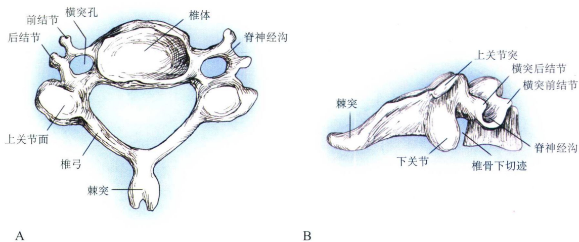
图 1-1-4 下颈椎
