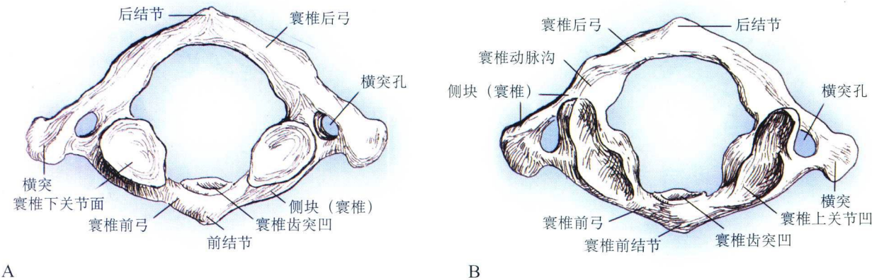
图 1-1-2 环椎
