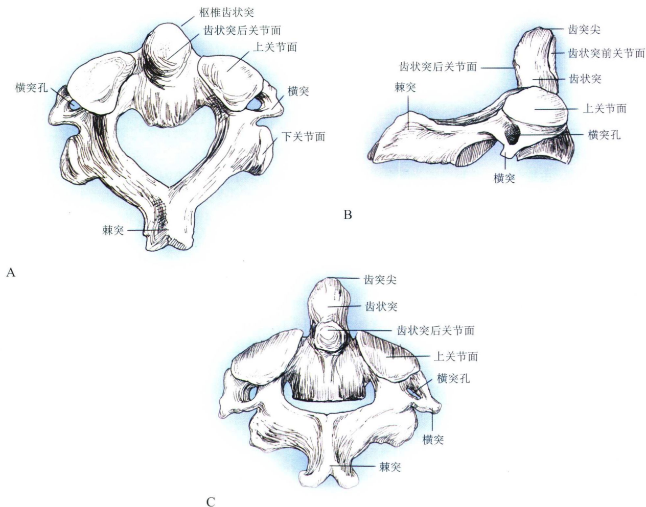
图 1-1-3 枢椎
