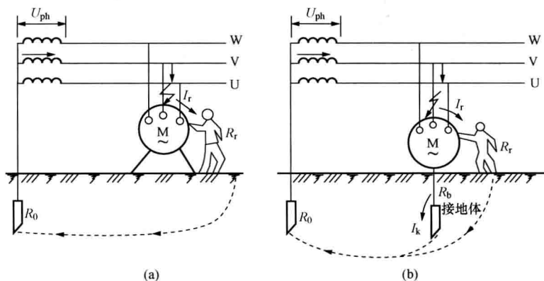
图 1-5 中性点接地系统保护接地原理
