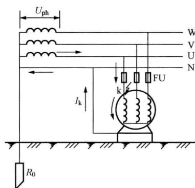
图 1-6 保护接中性线
