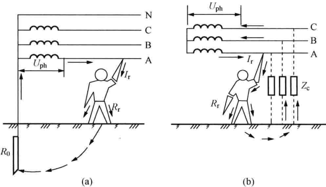
图 1 - 1 单相触电示意图 (a) 中性点直接接地系统的单相触电； (b) 中性点不接地系统的单相触电
