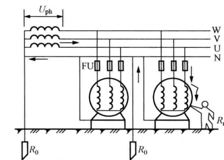
图 1-7 中性线的重复接地
