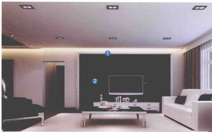
① 白枫木装饰线 ② 黑色烤漆玻璃
