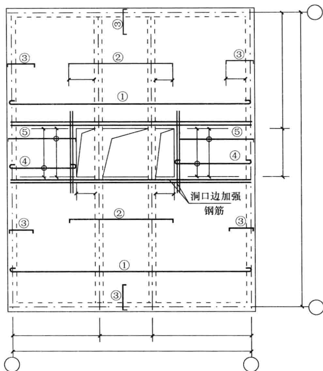
图 1-2 楼板配筋较复杂的表示方法
