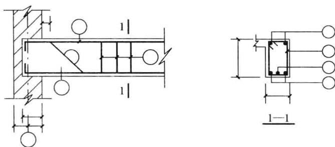
图 1-3 梁纵、横断面图中钢筋表示方法
