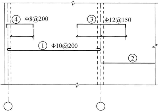
图 1-1 钢筋在楼板配筋图中的表示方法
