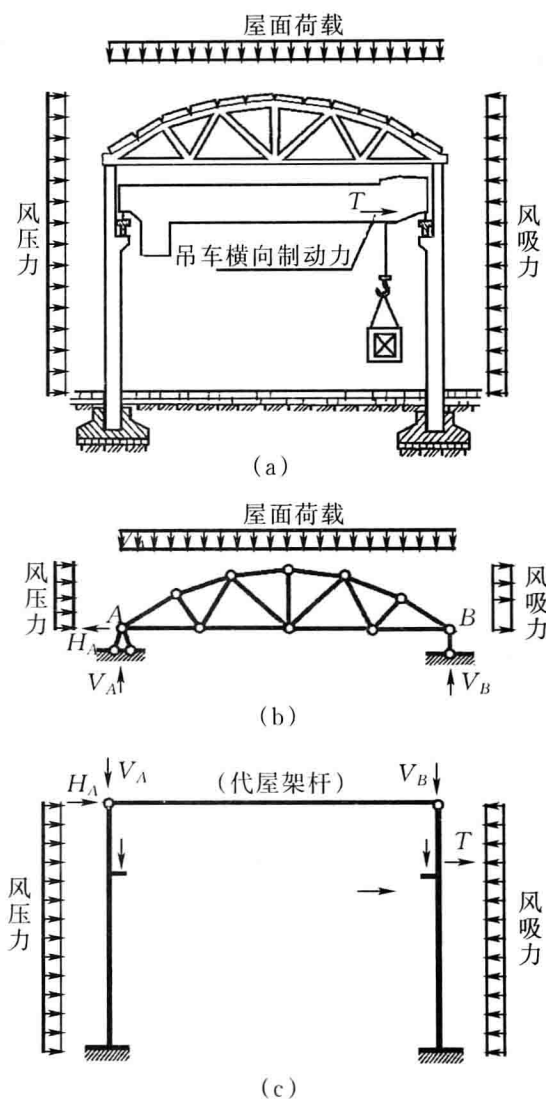
图 1-2 钢筋混凝土单层工业厂房计算简图
