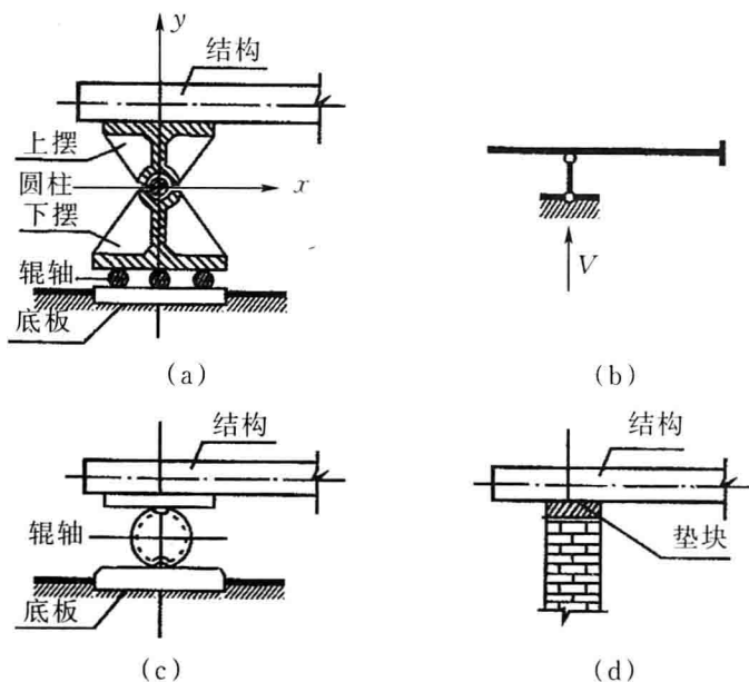
图 1-6 可动铰支座
