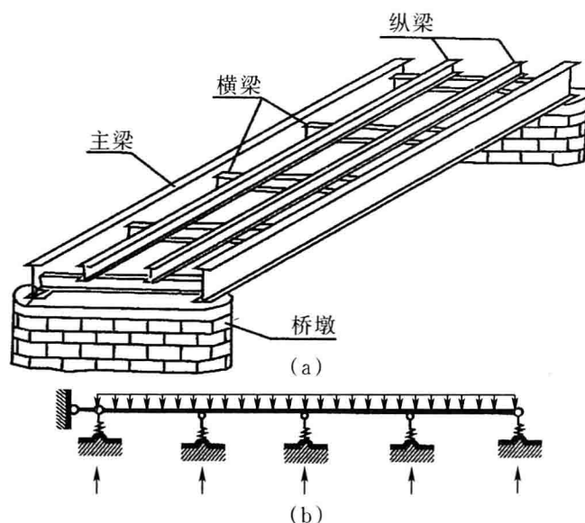
图1-10 伸缩弹性支座
