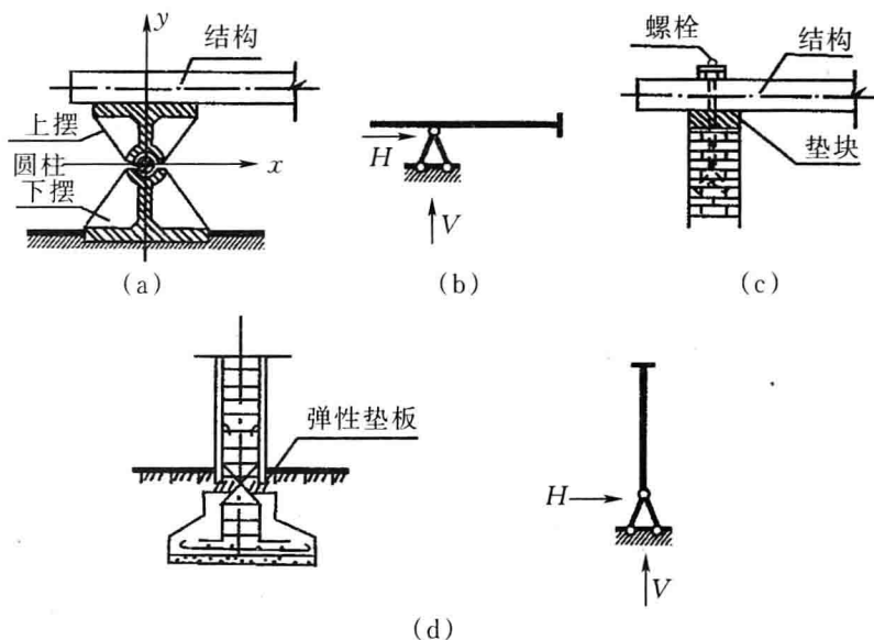
图1-7 固定铰支座
