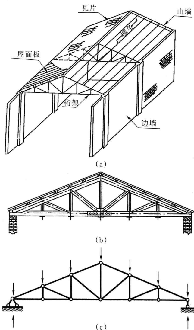
图1-1 砖木结构民用房屋计算简图
