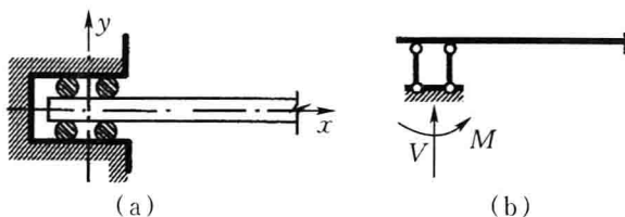
图1-9 定向支座
