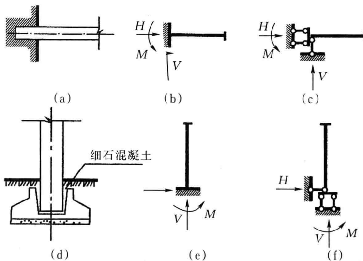
图1-8 固定支座
