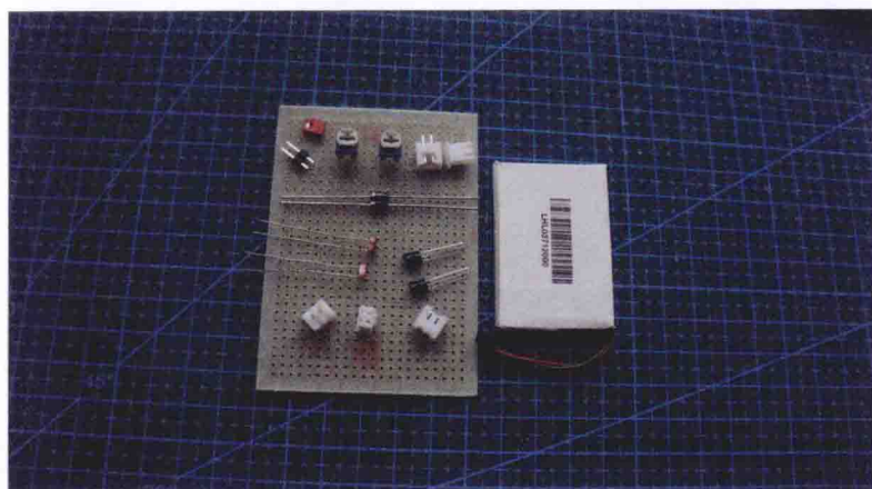
图1-8 机器人电子部分的主要元件。这里使用的三极管是C1815，可以替换成电流更大的8050，也可以使用其他型号的小功率NPN型三极管。锂电池充电器用一个报废的摩托罗拉手机充电器（标称输出4.4V/1A）改造而成
