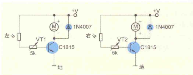
图 1-10 机器人电路图
