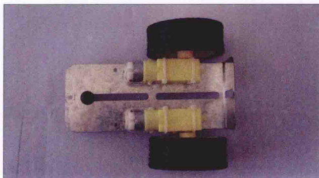
图 1-3 车体顶视图，左侧为车头。这是一个典型的双轮差速小车
