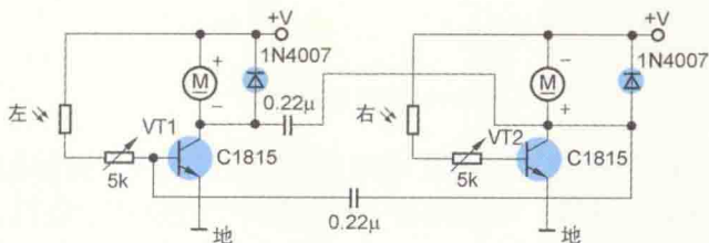
图 1-11 改进后的机器人电路图
