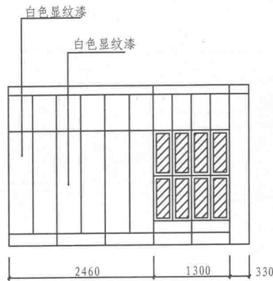
书房衣柜书柜图
