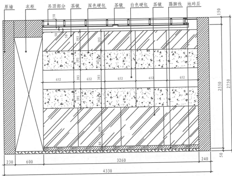
主卧背景墙立面图
