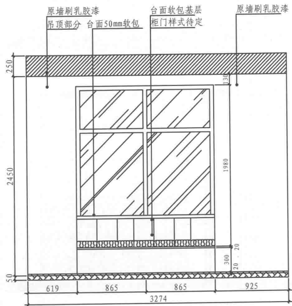
主卧飘窗立面图
