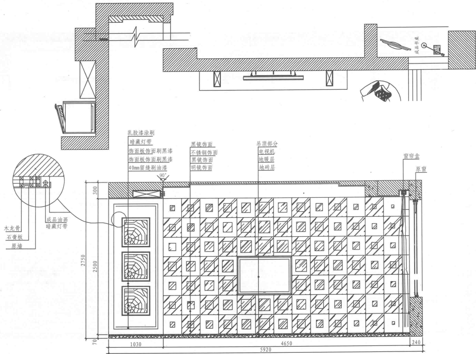
电视背景墙立面图
