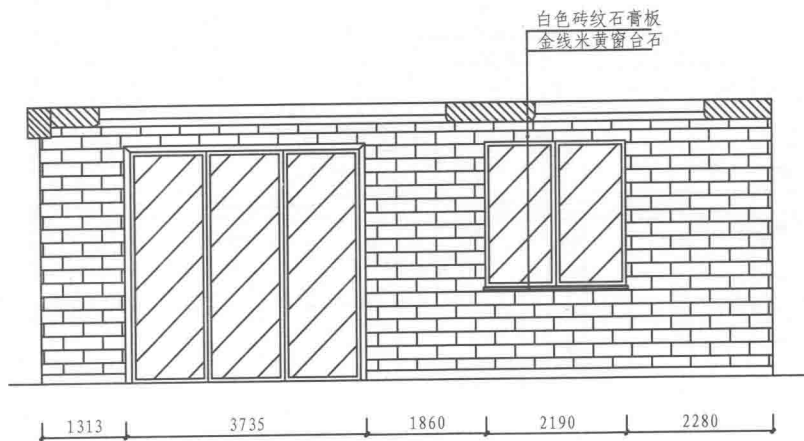
出阳台门立面图
