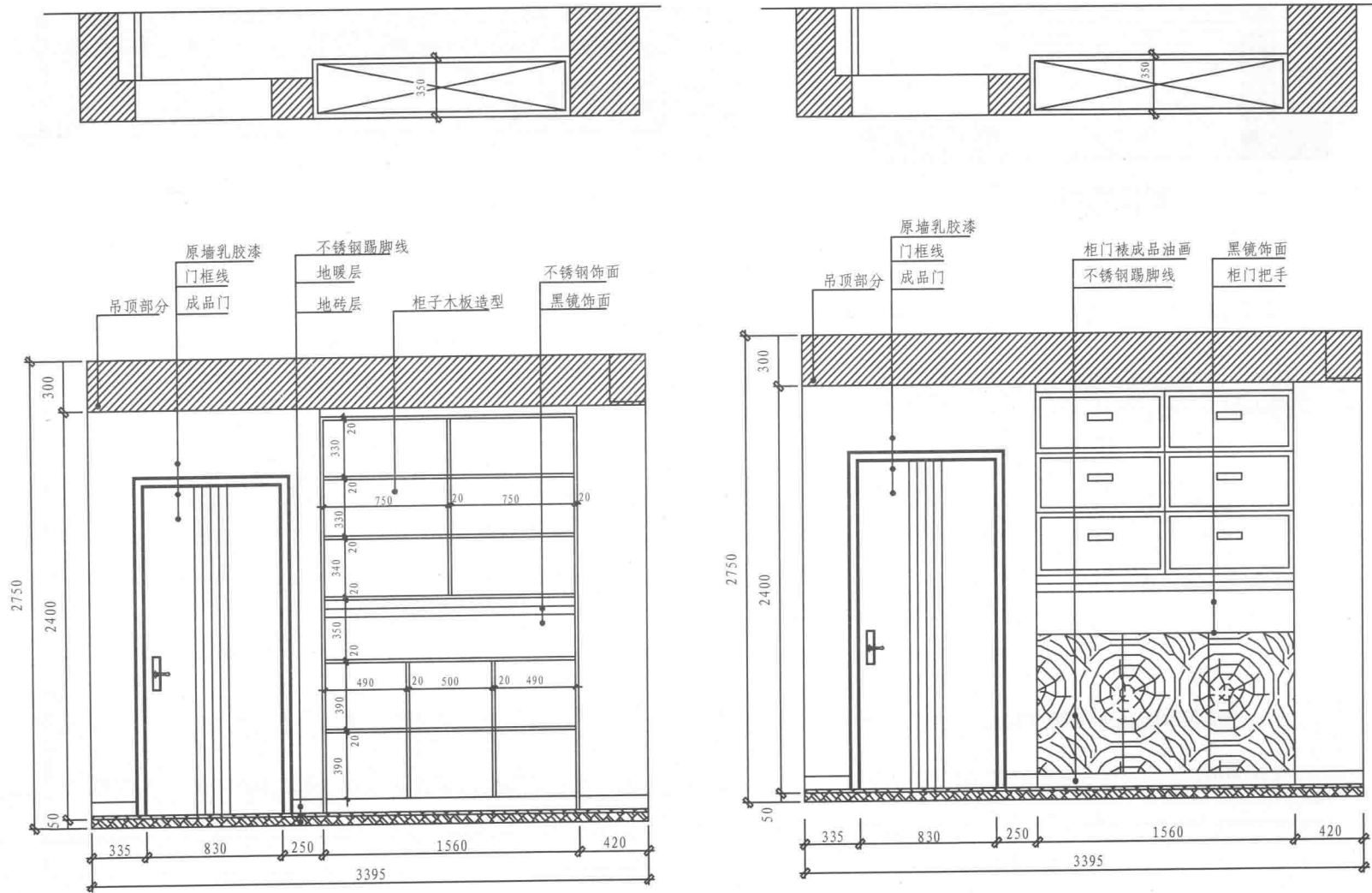
走道柜子立面图
