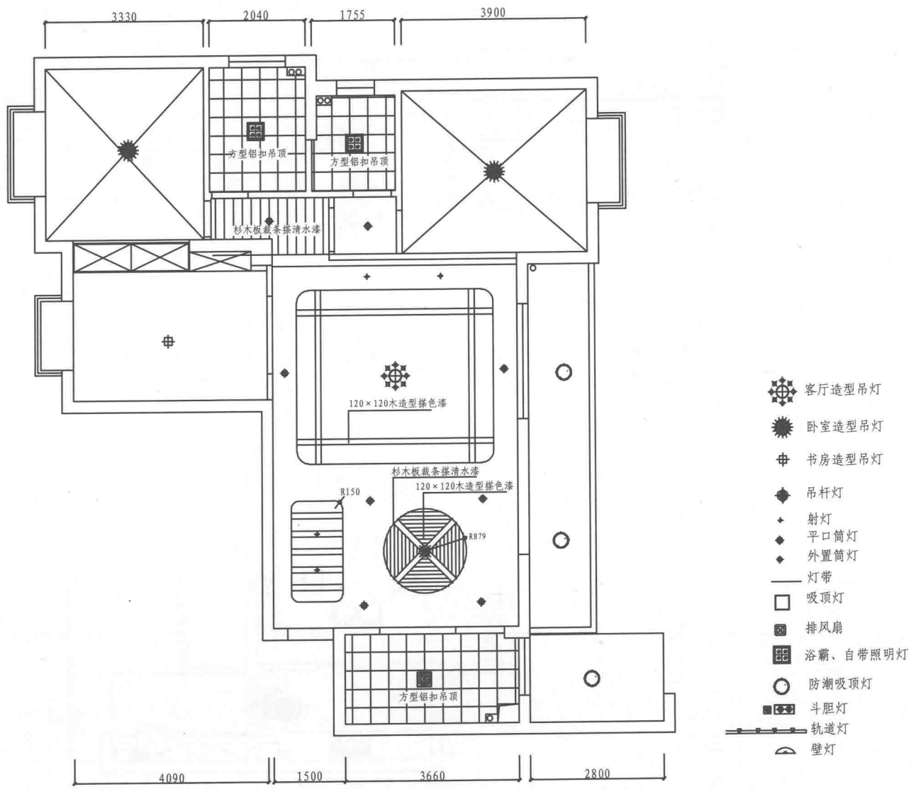
顶面布置图
