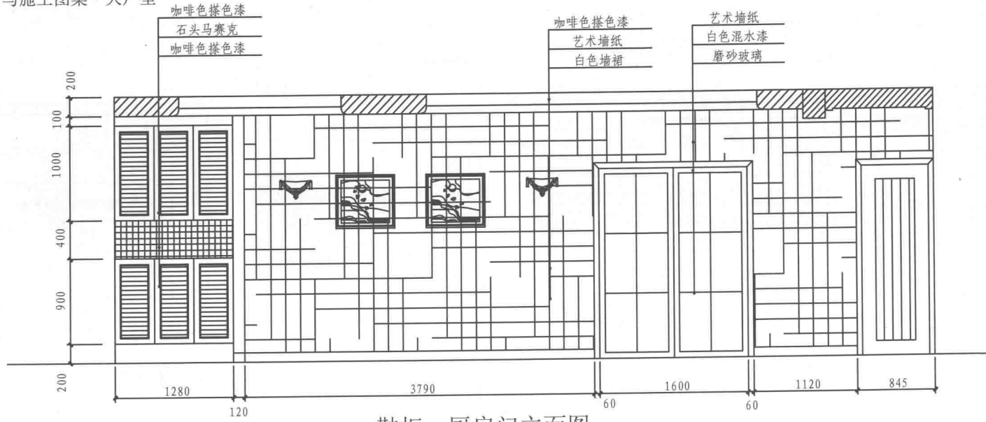
鞋柜、厨房门立面图
