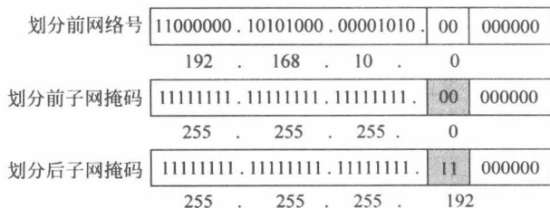
图 1-3 子网划分前后的子网掩码
