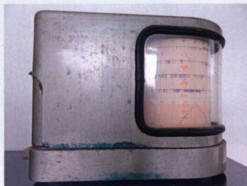
EL 型电接风风向风速自记仪
