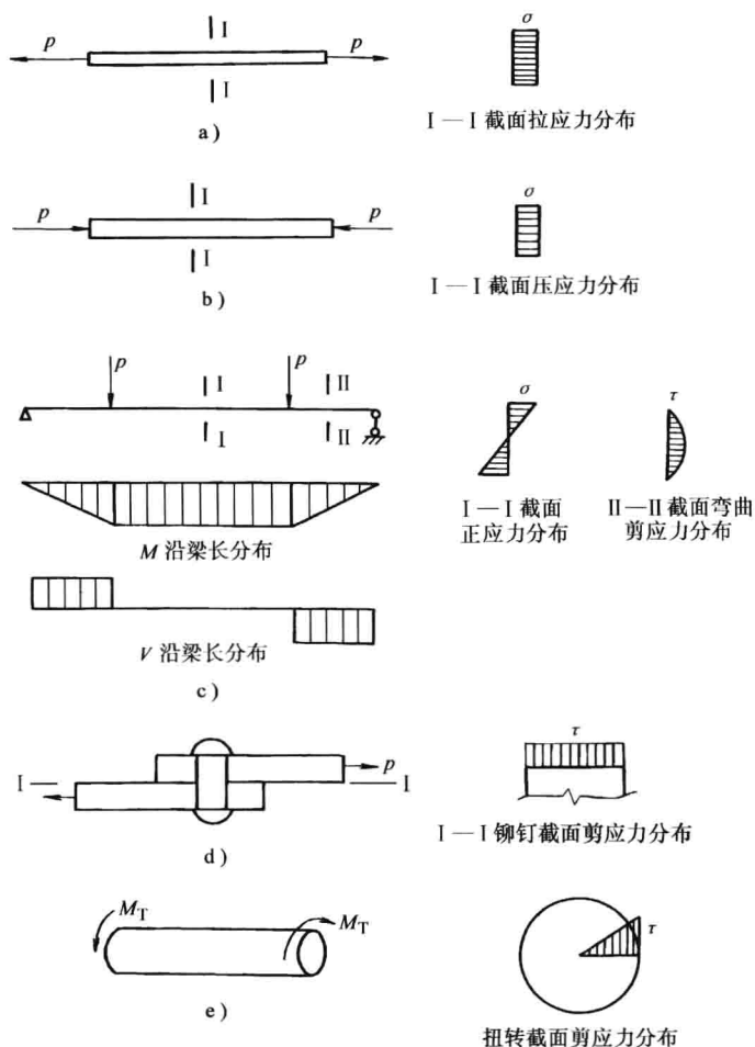
图 1-1 构件基本受力状态
