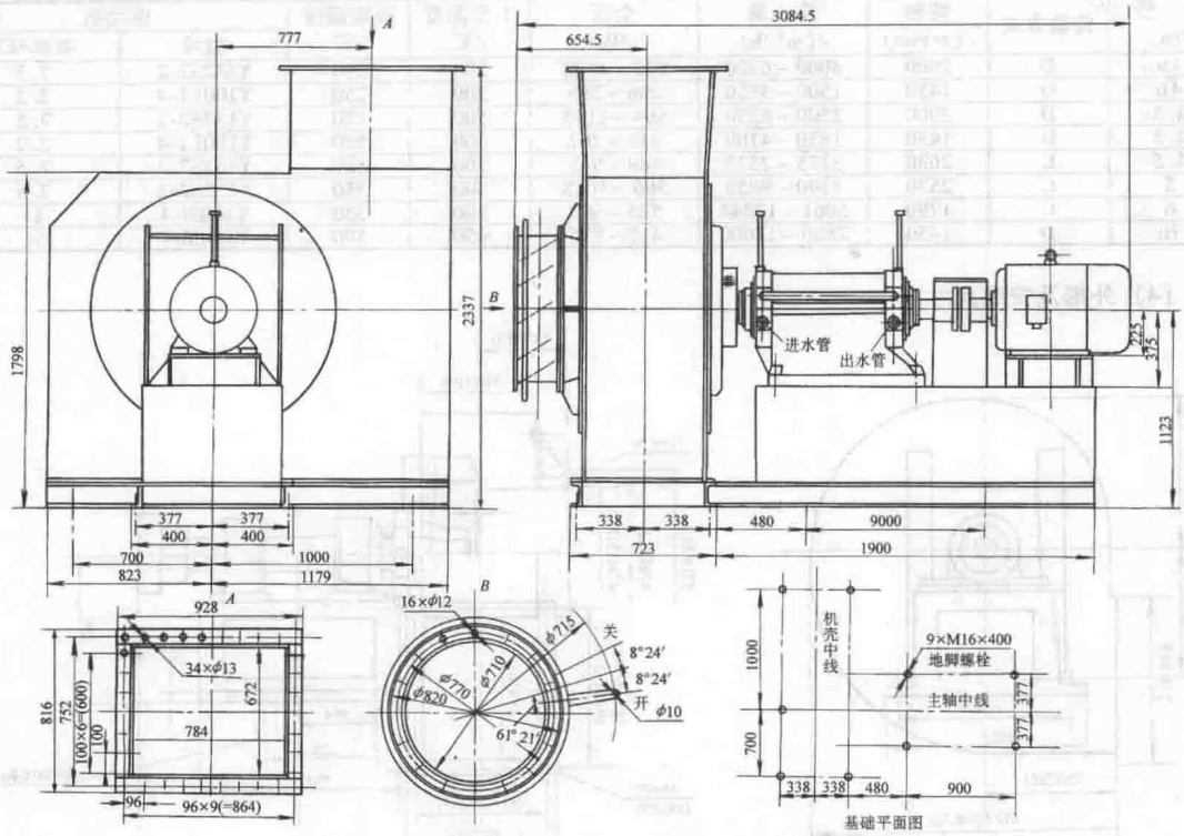
W4-57-11No. 11. 2D (逆 90°) 离心通风机的外形及安装尺寸
