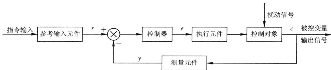
图 1-2 室温控制系统功能框图
