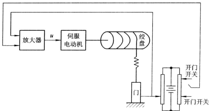
图 1-6 仓库大门自动控制系统
