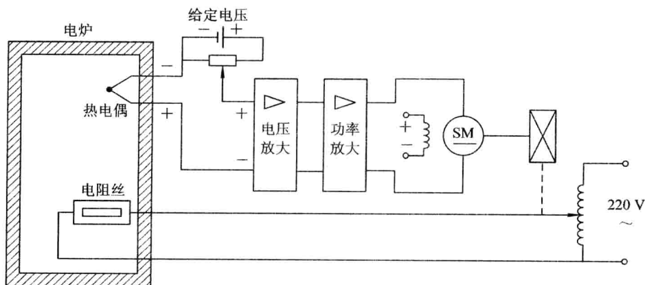
图 1-7 电炉温度控制系统
