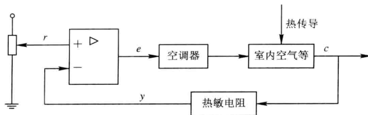
图 1-1 室温控制系统元部件框图
