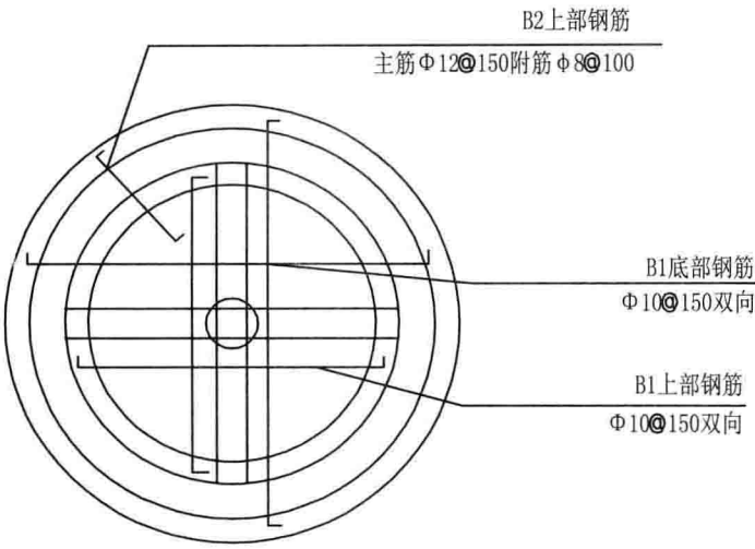
结构平面图
