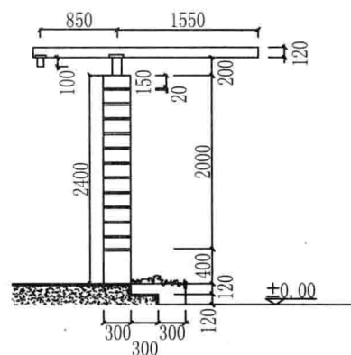
大样图
