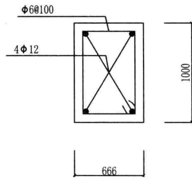
3-3剖面图
