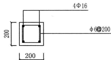
L1剖面图
