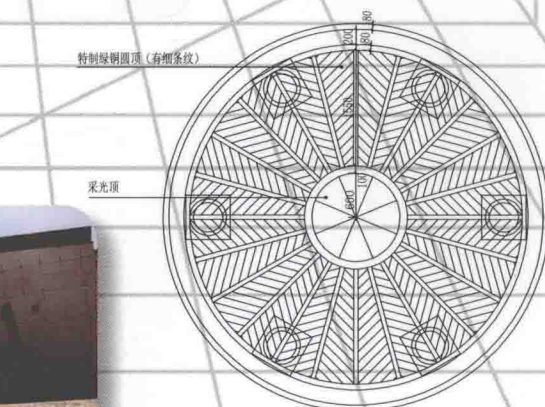
顶平面图
