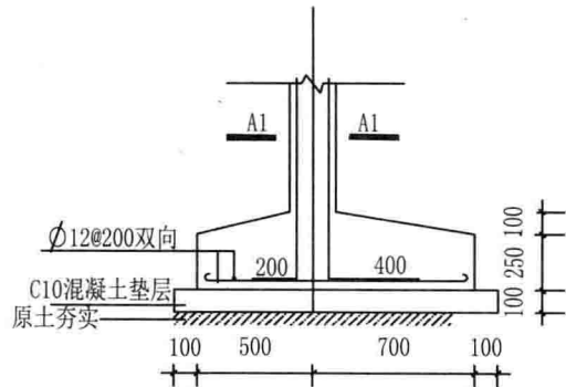
C-C剖面图
