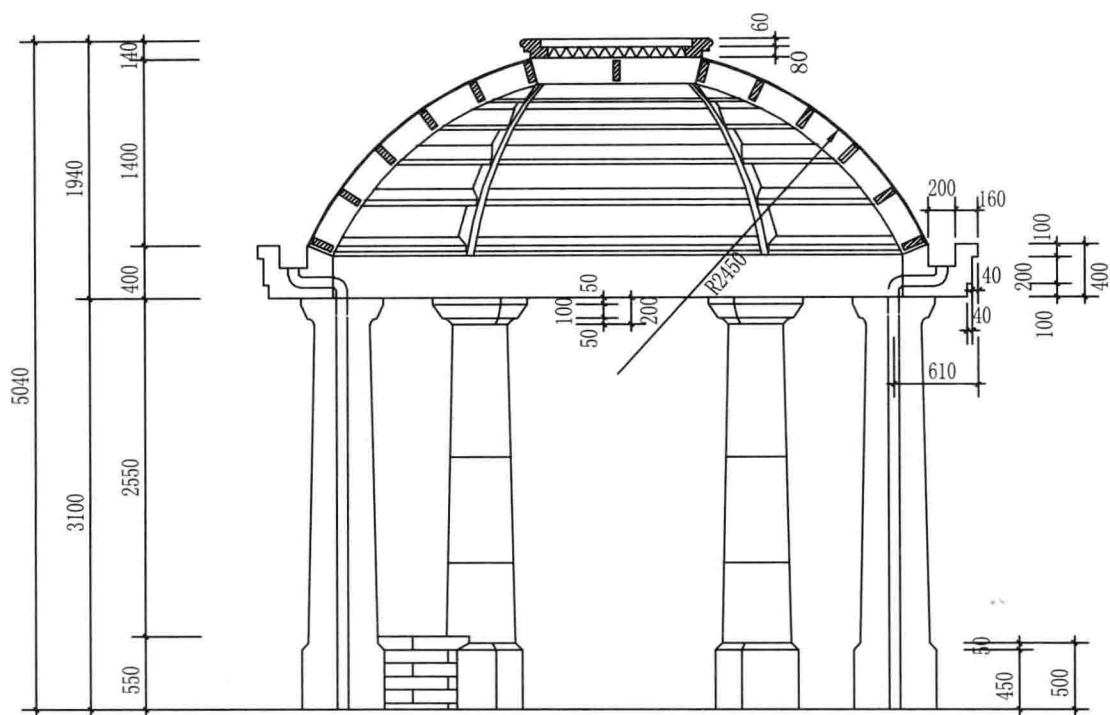
剖面图
