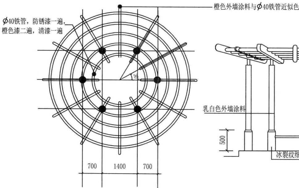
俯视平面图
