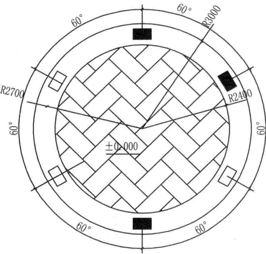
平面图
