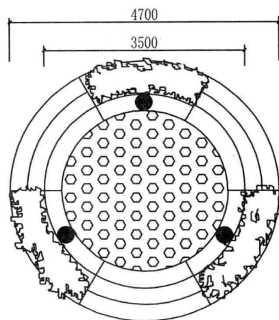
底平面图
