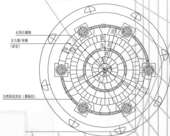
底平面图
