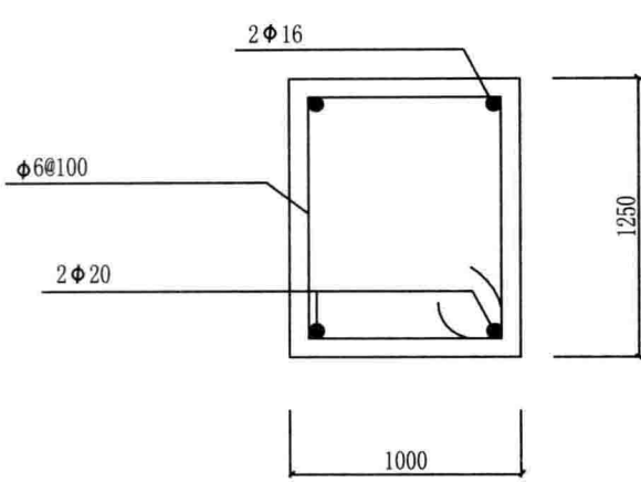
1-1剖面图
