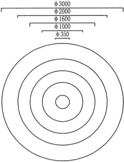
顶面平面图
