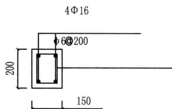
L2剖面图
