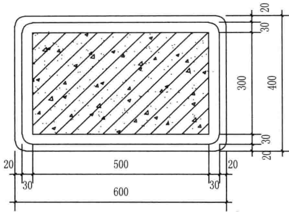
1-1剖面图
