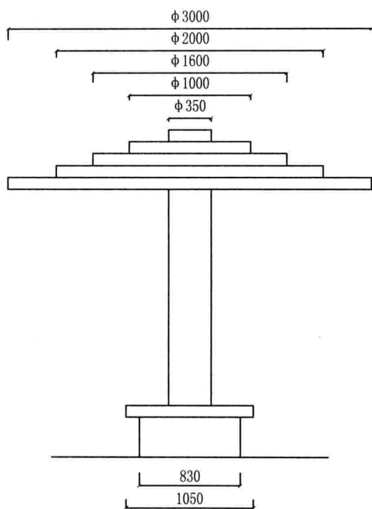
立面图
