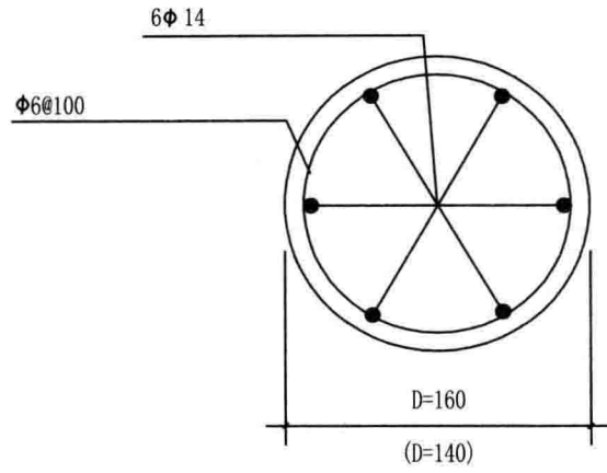
A1-A1 (A2-A2)剖面图
