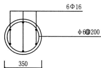
柱剖面图
