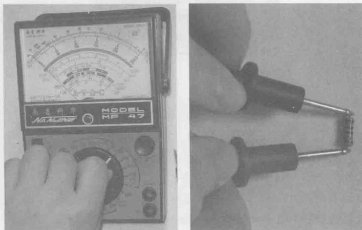
图 1-5 指针式万用表测量电阻示范图
