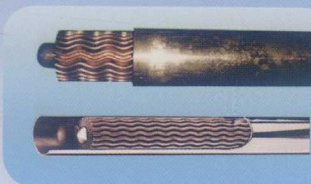
内翅片换热管
