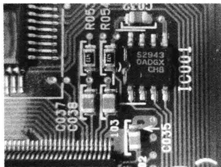
12 代皇冠智能钥匙 ECU 板存储芯片 S2943
