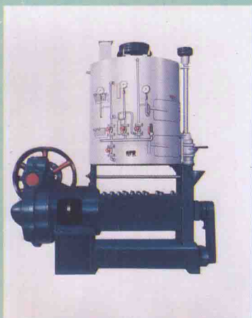
该图片为保定地区棉油机械厂产品 200A-3型螺旋榨油机
