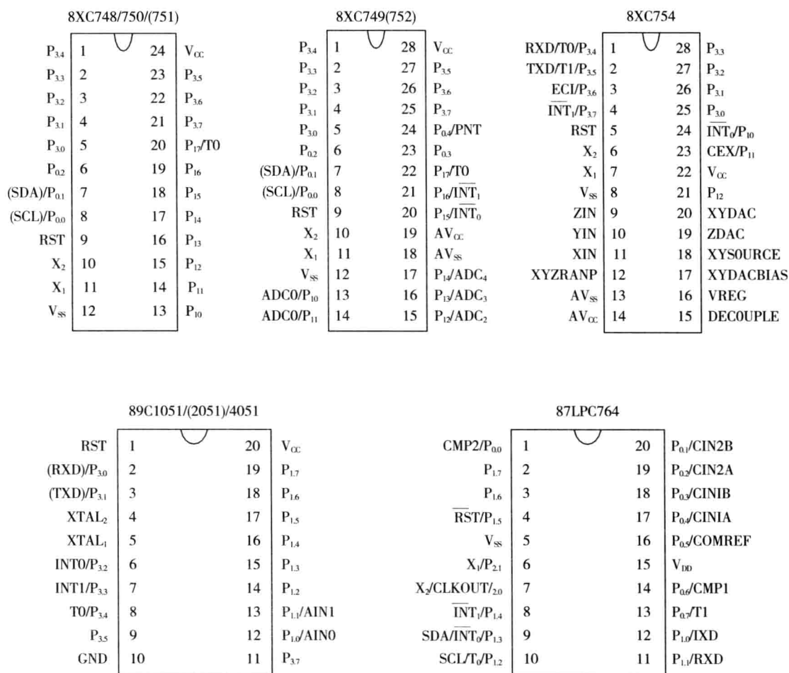
图 1-1 80C51 系列非总线型单片机
