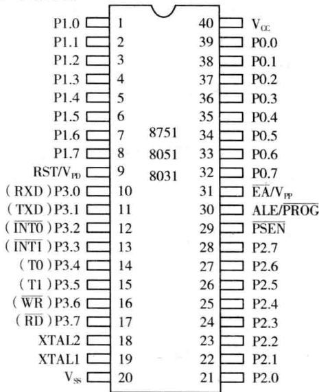
图 2-3 MCS-51 双列直插封装方式的引脚
