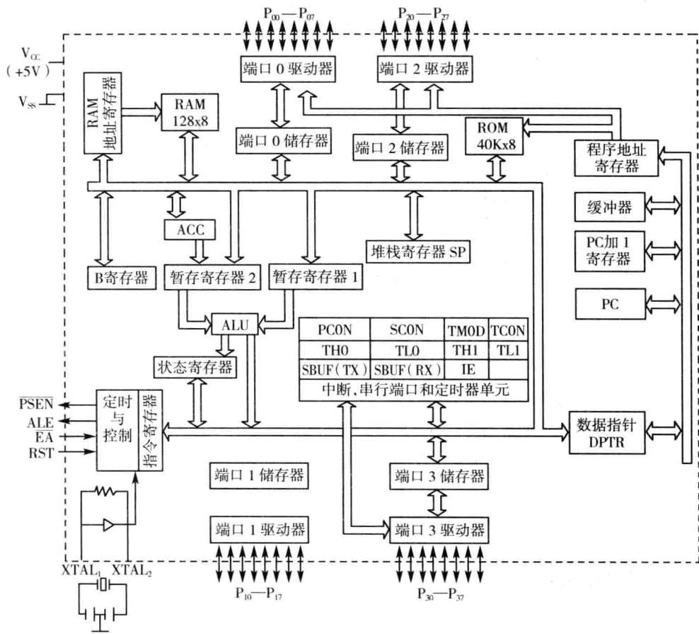
图 2-2 8051 内部结构框图
