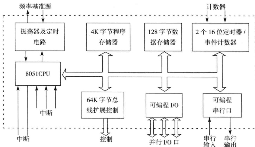
图 2-1 8051 单片机框图
