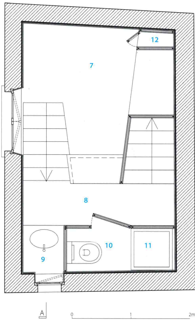
阁楼平面图
