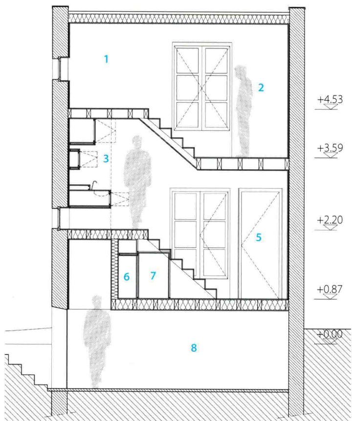
剖面图AA
