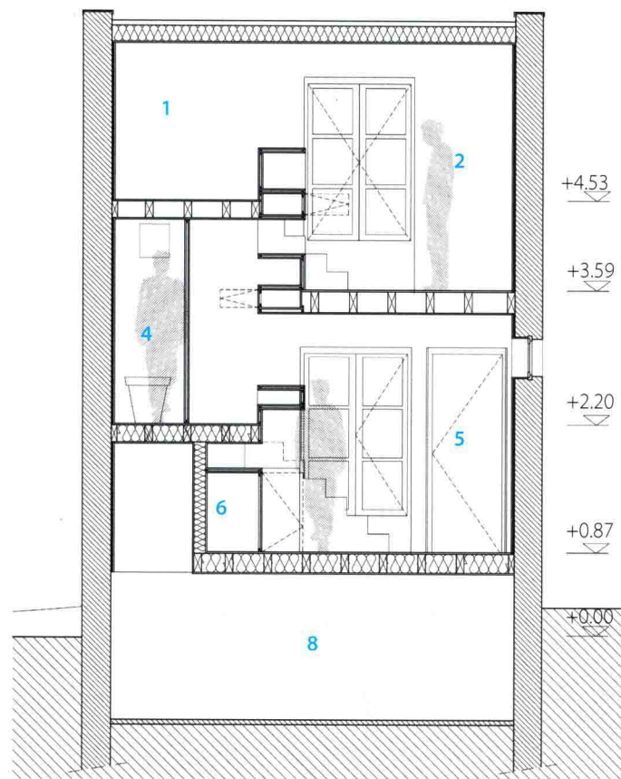
剖面图BB
