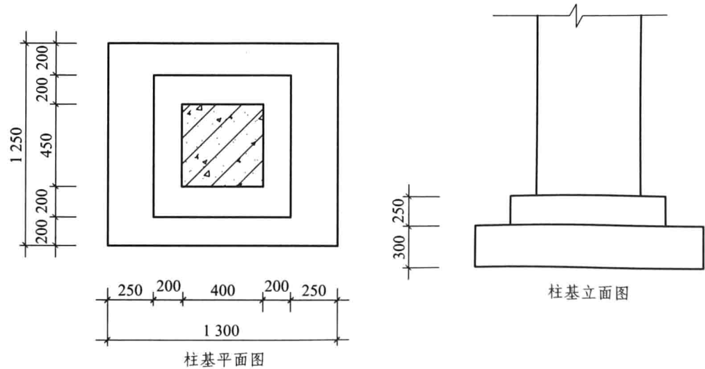
图 1.1 现浇独立基础
