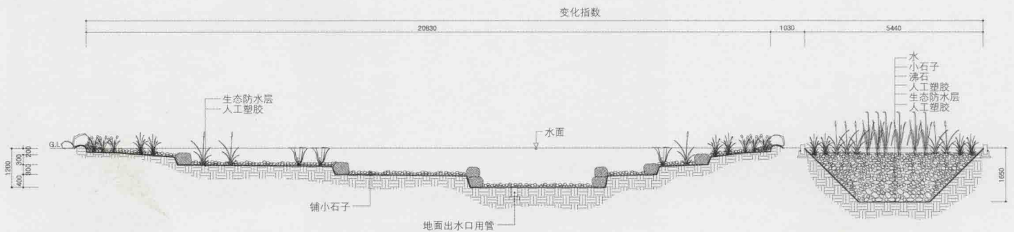
水景剖面图
