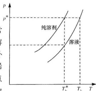
图 1-1 稀溶液的沸点升高
