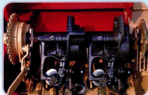
关键部件——打结器，为德国原装进口件，保证了打捆机高成捆率
