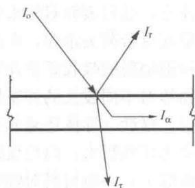
图 17-2 物体对外来辐射的反射、吸收和透射
