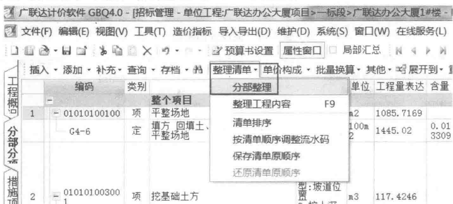
图 2.9 选择“分部整理”功能
