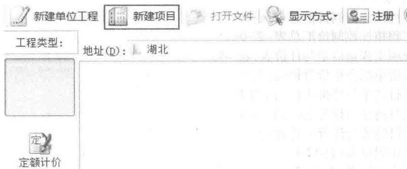
图2.1 新建项目
