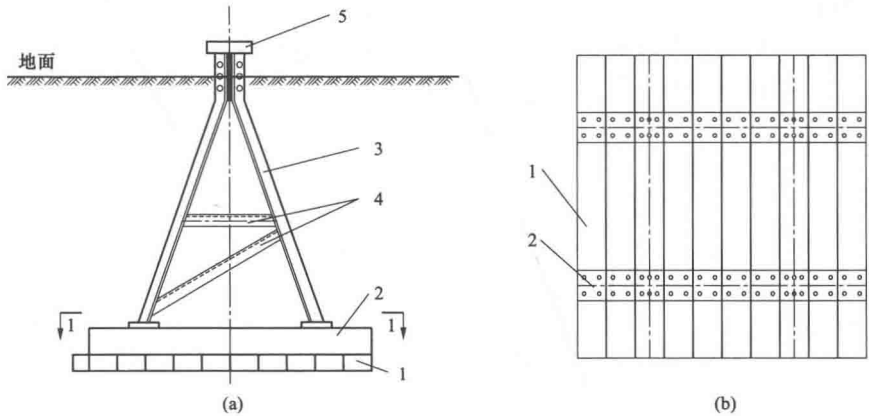
图 1-5 混凝土板条和金属支架组合而成的装配式基础 (a) 基础组装图；(b) 1-1 剖面图
