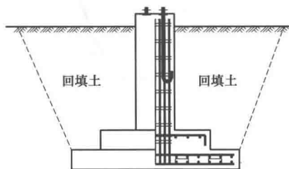
图 1-2 直柱柔性板式基础
