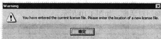
图 1.14 警告对话框
