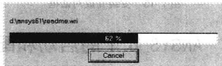
图 1.11 安装进度条
