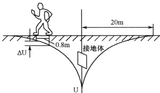
图 1-1-1-3 跨步电压触电
