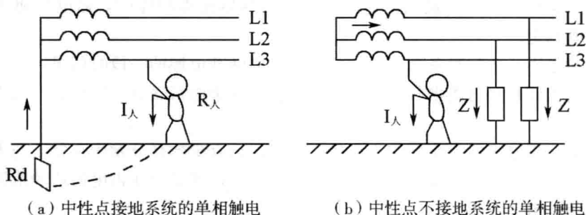
图 1-1-1-1 单相触电
