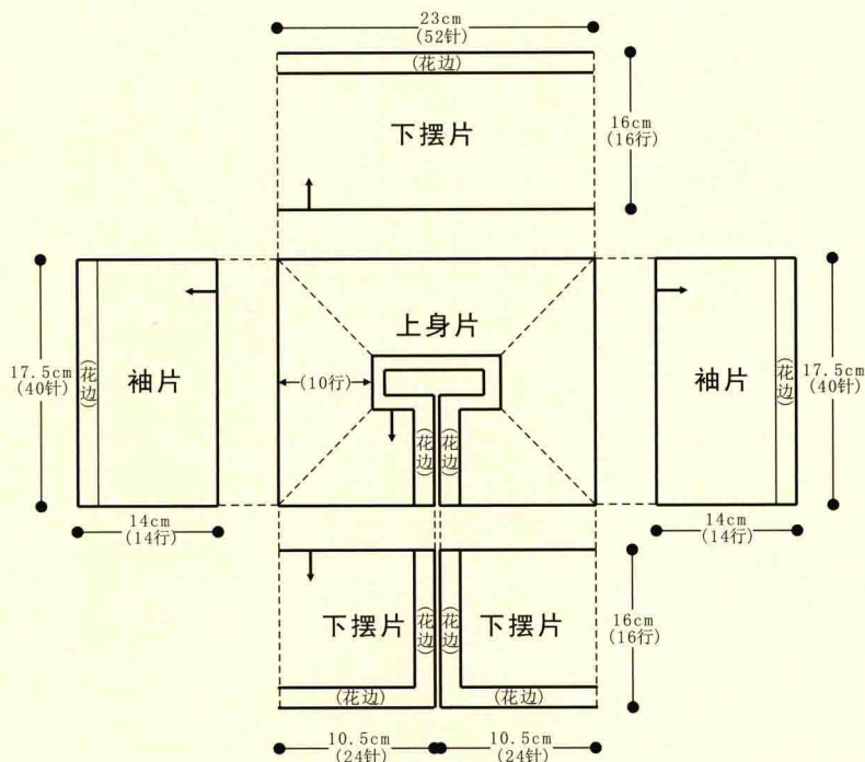
上衣结构图
