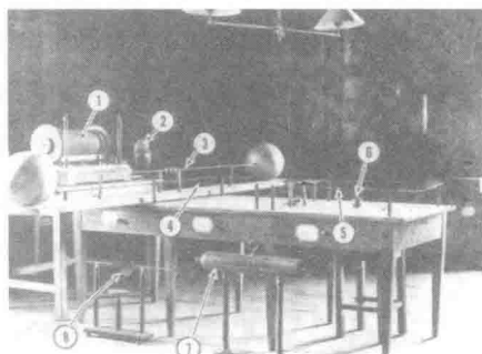
图1.1 赫兹的装置及简图（Schleiermacher 1901）
