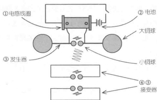
图1.1 赫兹的装置及简图（Schleiermacher 1901）
