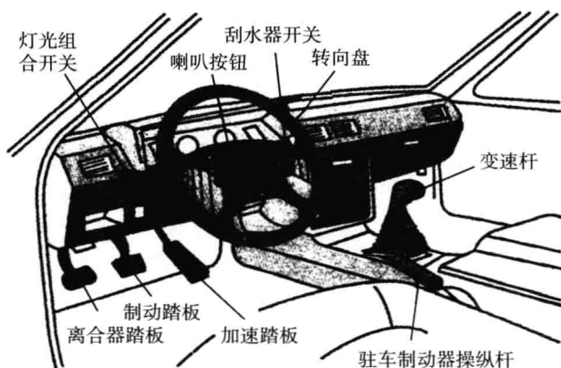
图1-1 手动挡汽车驾驶操纵装置
