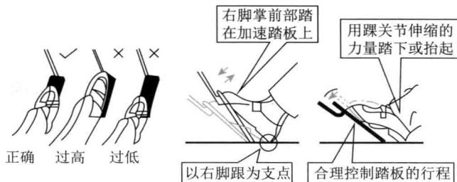
图1-5 加速踏板
