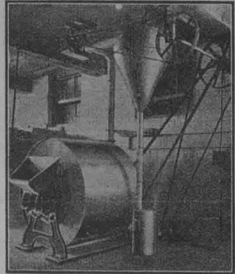
美國茶葉混合機，附有空氣吸引裝置
