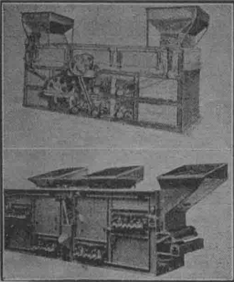
英國一六——軸碎切篩分機
