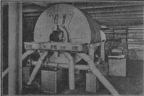
波士頓UMBO式旋轉茶葉混合機
