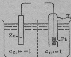
图 1-1. 鋅电极与氢电极組成的化学電池。
