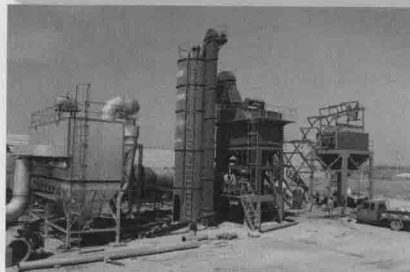
沥青拌合机除尘设备系列产品 XMC 脉冲袋式除尘器系列(适用于 1000-4000 型)
