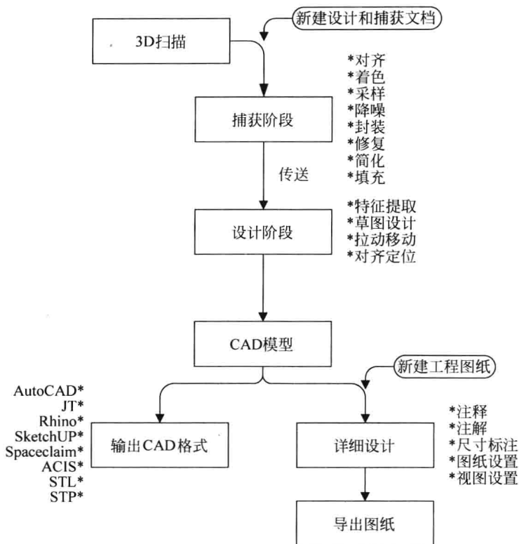
图 2-1 Geomagic Design Direct 混合建模基本流程
