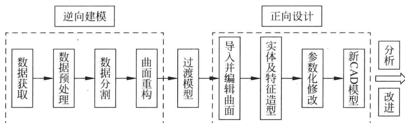
图 1-3 混合建模一般流程
