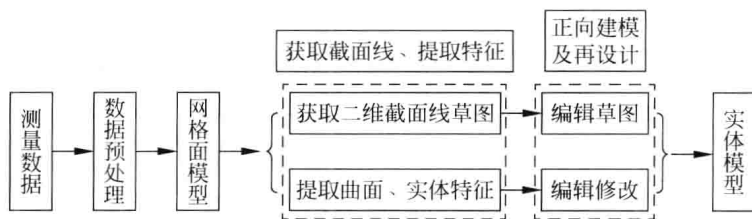
图 1-4 Geomagic Design Direct 混合建模流程
