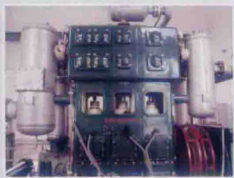
2000-2400m³/h 系列氧气压缩机 200-2400m³/h Series Oxygen Compressor
