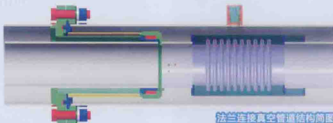
法兰连接真空管道结构简图
