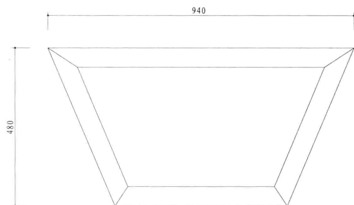
俯视图
