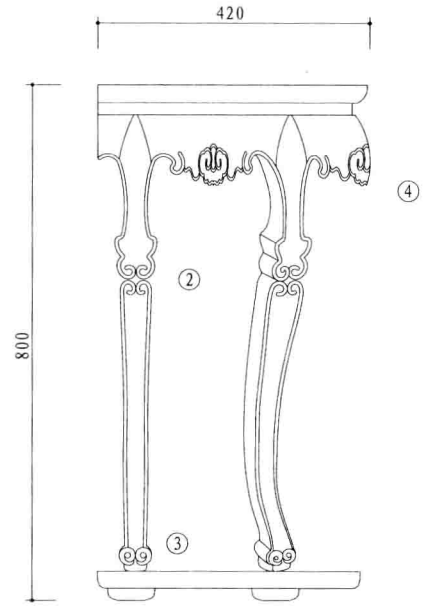
左视图
