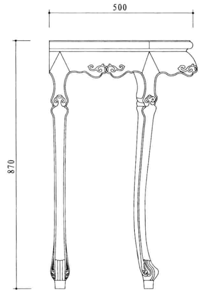
左视图
