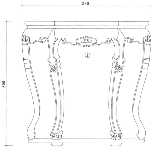
主视图
