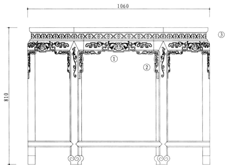
主视图
