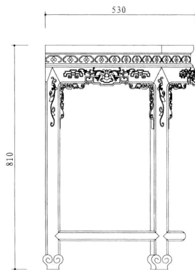
左视图
