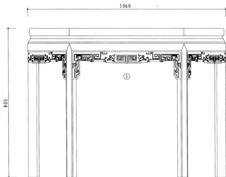
主视图
