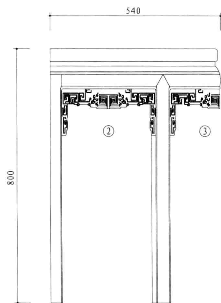
左视图
