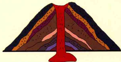
火山渣锥
