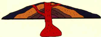
盾火山
