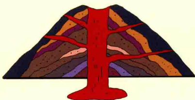
层火山
