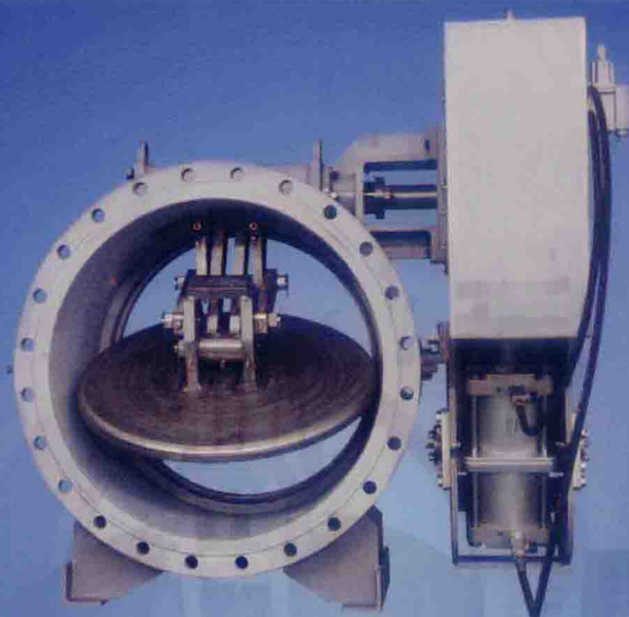
分子筛纯化系统用三杆阀
