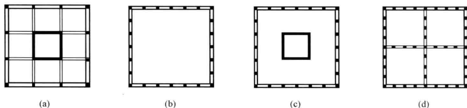
图 1-1 筒式体系的形式
