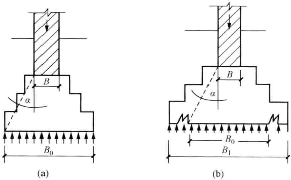
图 1-3 刚性基础受力特点
