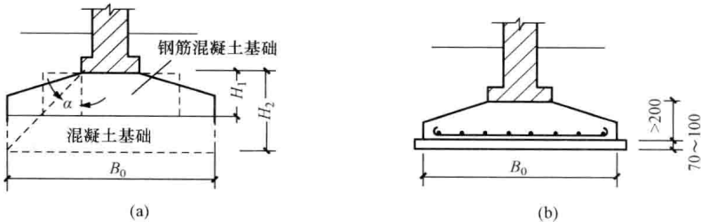
图 1-4 钢筋混凝土基础
