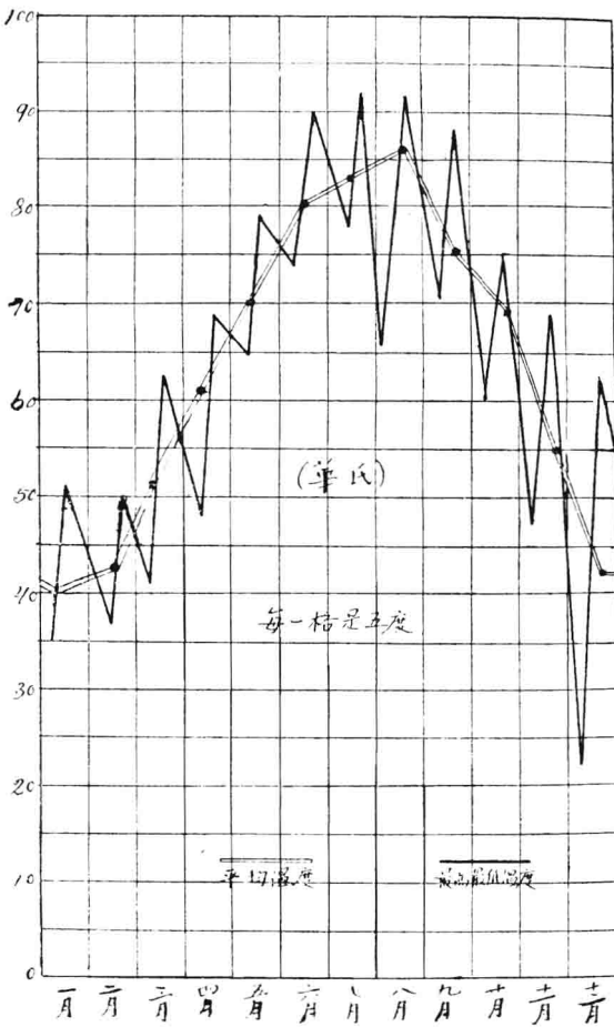
无锡县十八年温度升降表
