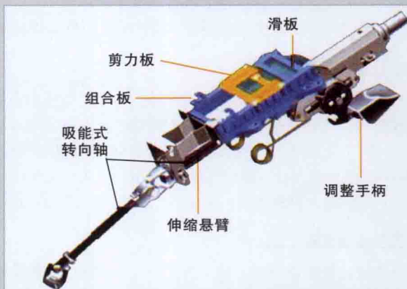
图1 转向管柱伸缩机构
