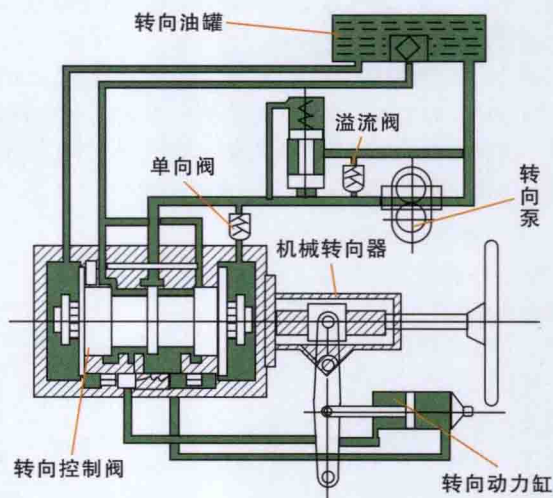
图1 常流式液压动力转向系统示意图
