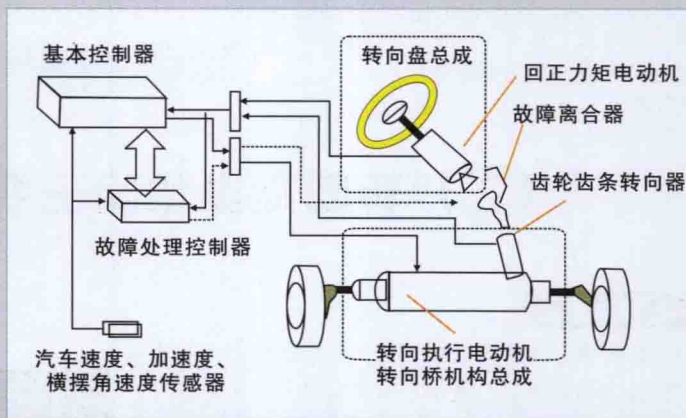
图2 汽车线控转向系统结构
