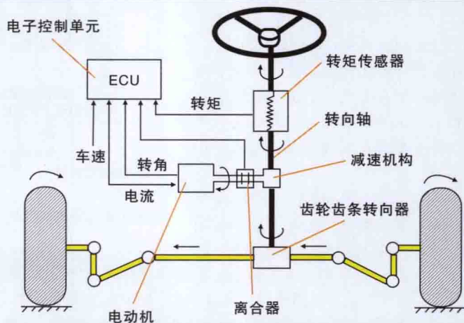
图2 直接助力式电动转向系统示意图
