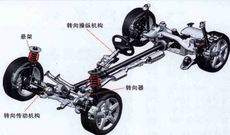
图1 转向系统的组成部分
