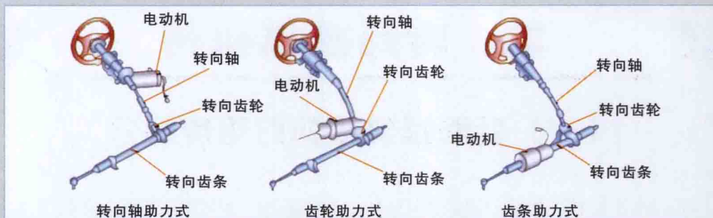
图1 直接助力式电动转向系统类型
