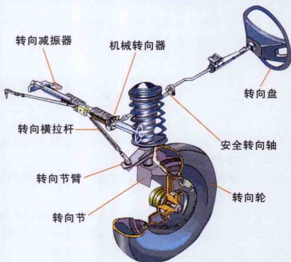
图2 机械转向系统（红旗CA7220型轿车）
