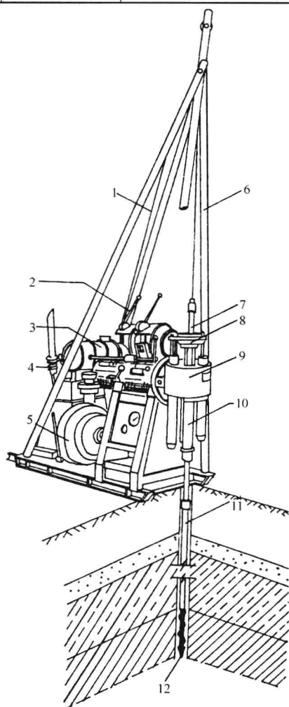
图 1-1 SH-30 型钻机结构示意图
