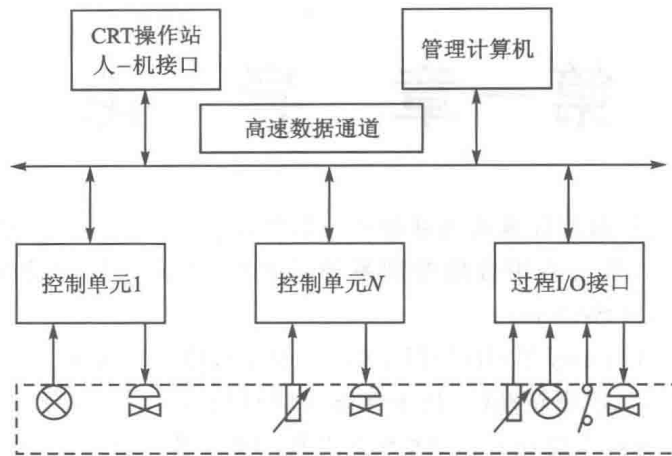
图 1.1 集散型控制系统基本结构
