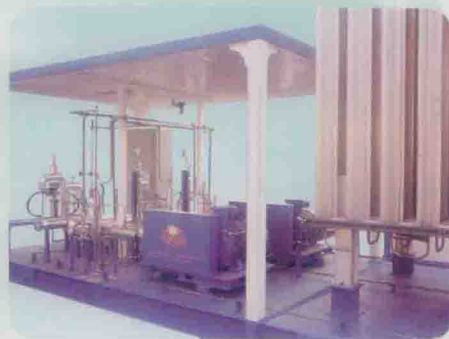
L-CNG 汽车加注撬
