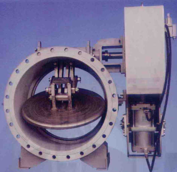
分子筛纯化系统用三杆阀
