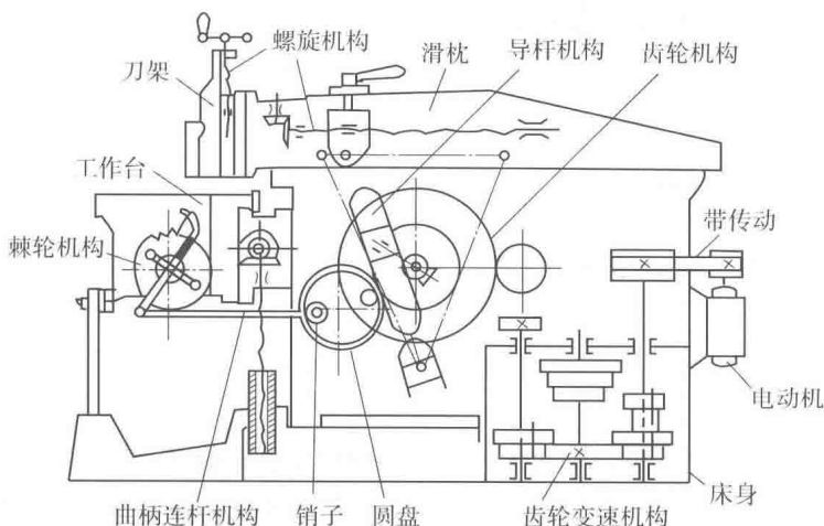
图 1-2 牛头刨床的传动系统
