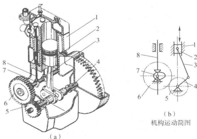
图 1-3 内燃机
