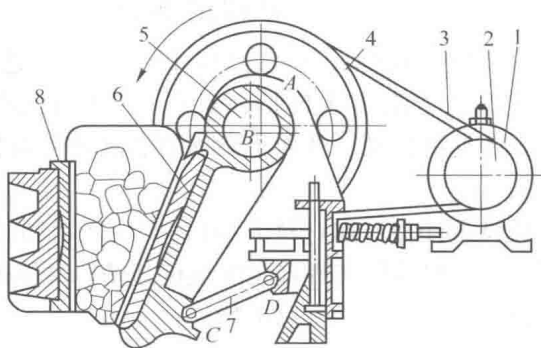
图 1-1 颚式破碎机
