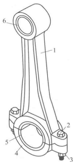
图 1-4 内燃机连杆
