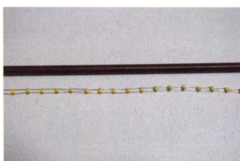
11 焊好燈帶後，其長度要跟膠管長度相同（14.5cm）。
