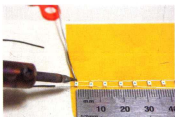
10 用焊錫器將錫線、LED燈及鍍電線焊在一起。
