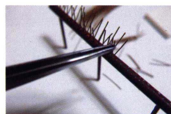
21 在已鑽孔的位置，植入已裁好的光纖線。
