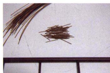
19 將光纖線裁切成8mm至15mm長。
