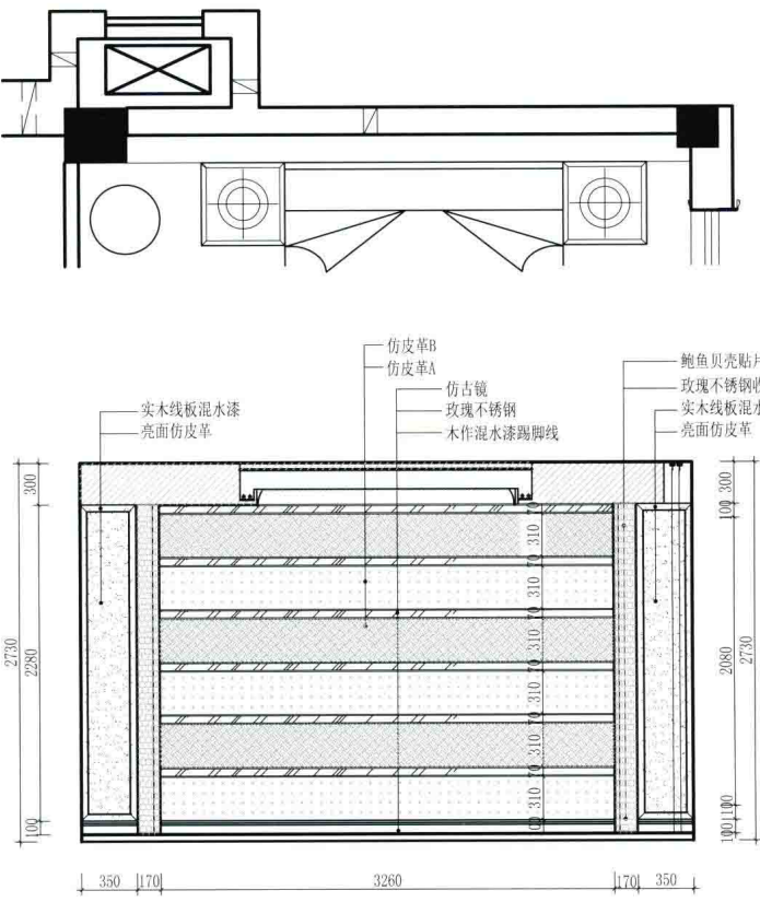
三层主卧立面图
