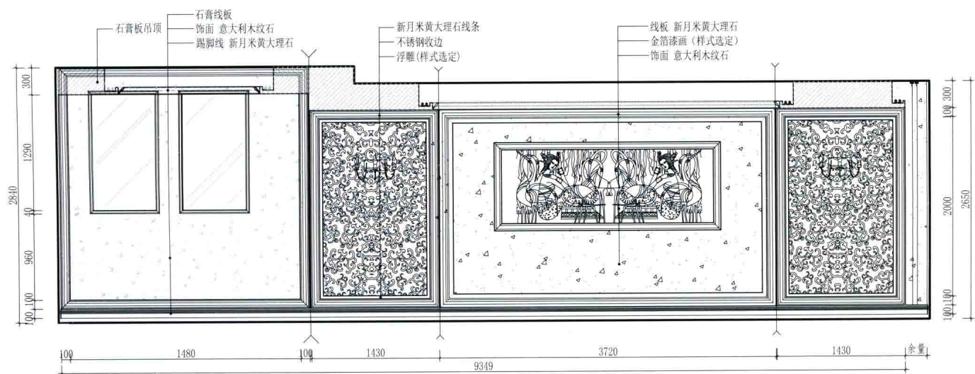
一层客厅立面图
