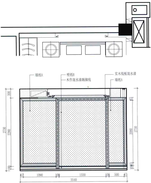
儿童房立面图
