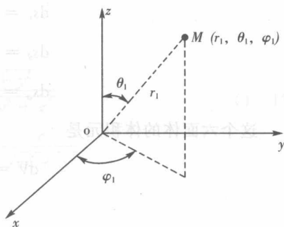
图 1-5 球坐标系
