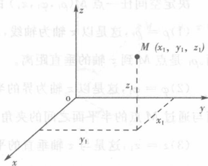
图1-1 直角坐标系
