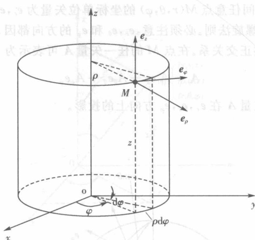
图 1-4 柱坐标系的单位矢量
