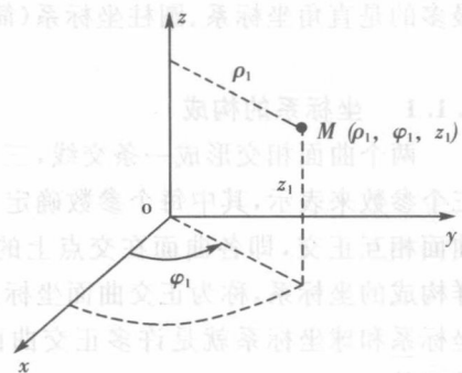
图 1-3 柱坐标系
