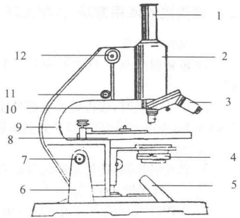
图 1-1 显微镜结构图
